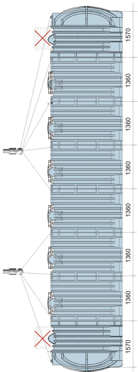
Рисунок 10. Схема строповки нескольких емкостей (40000 литров)
