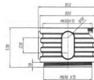
Рисунок 5. Чертеж горловины
