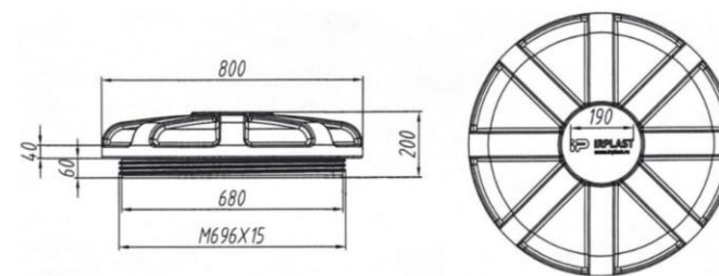
Рисунок 6. Чертеж крышки
