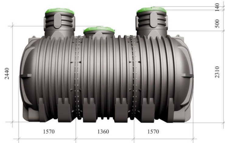
Рисунок 2. Модули резервуара
