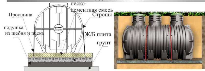
Рисунок 13. Схема установки подушки под плиту основание
