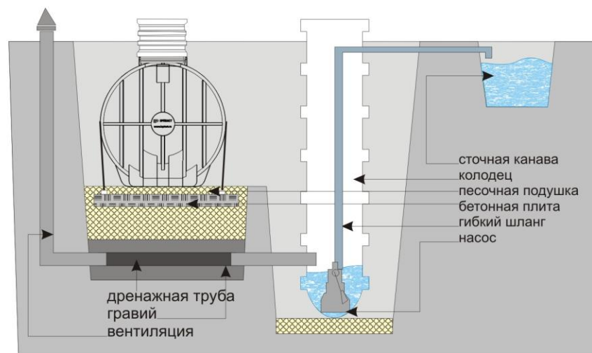
Рисунок 15. Схема дренажа
